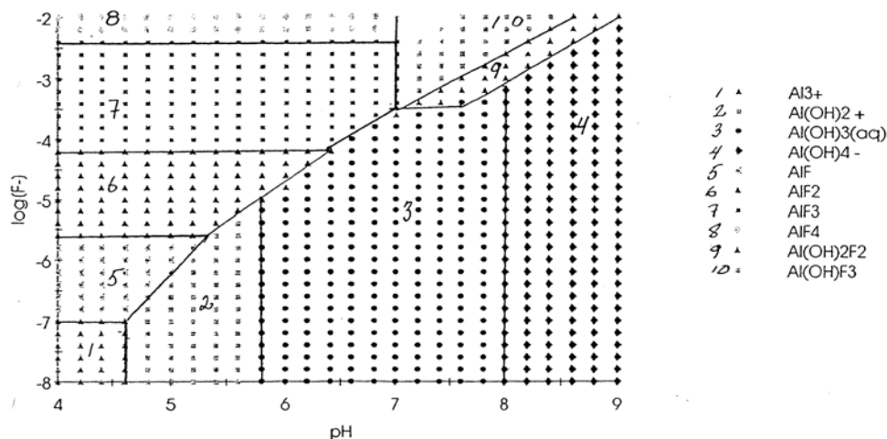
Figure 1.1. Predominance area diagram of the \text{Al}^{3+} -F-OH- system (Sjöberg, 2002)
