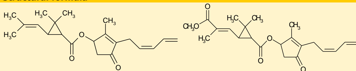
pyrethrin 1
