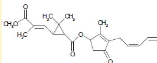
pyrethrin 2
