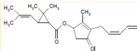
pyrethrin 1
