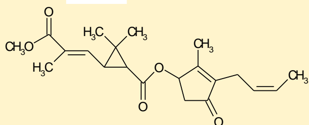
cinerin 1
