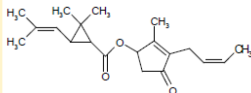
pyrethrin 1
