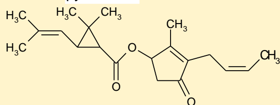
pyrethrin 1
