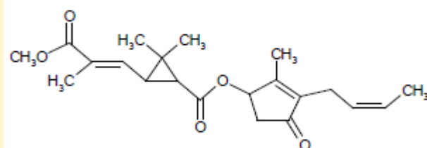
pyrethrin 2
