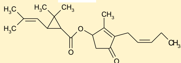
cinerin 2
